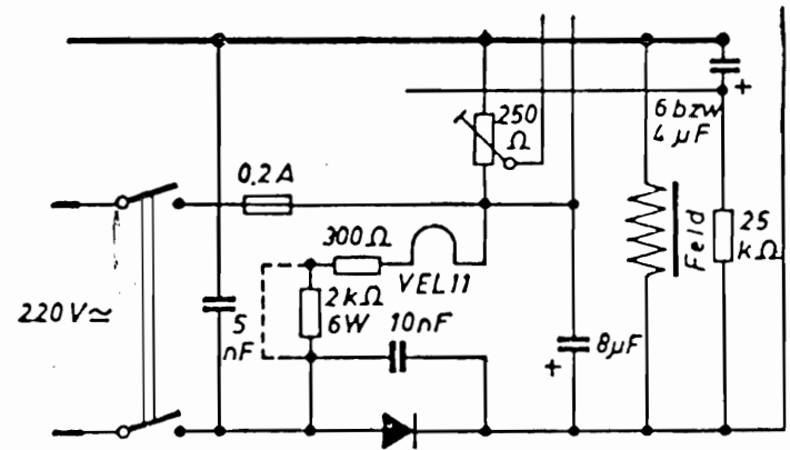
Netzteil für Ausfg. II
